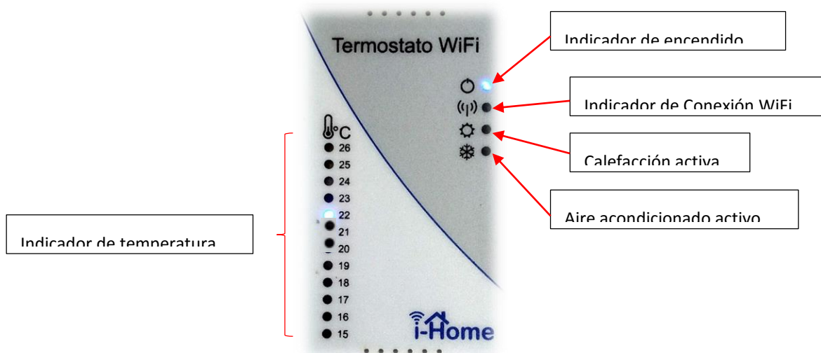
Ilustración 30: Vista del panel frontal
